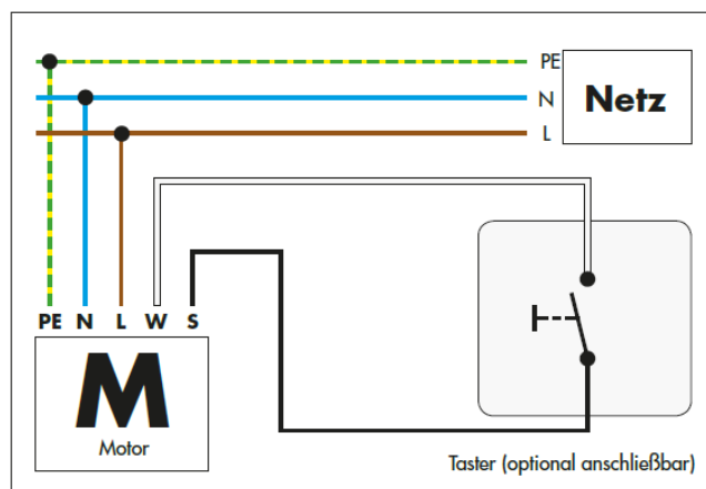
Abb.2: Anschlussschema Art. 140010 - 140050
