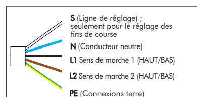
Fig. 3 Connexion du moteur avec l'interrupteur des stores
