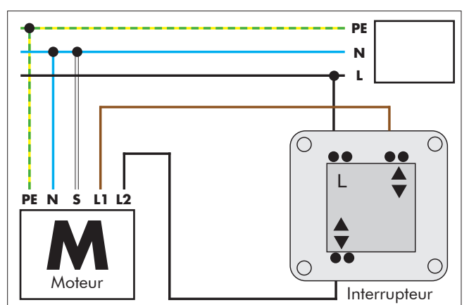
Fig. 3 Connexion du moteur avec l'interrupteur des stores
