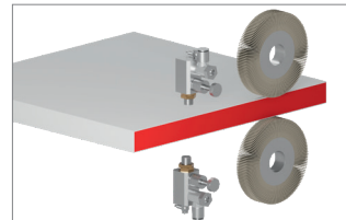
4 zóna pro dokončovací práce
